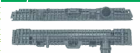
11725 / Axor superior (c/ retorno) (modelo valeo)
