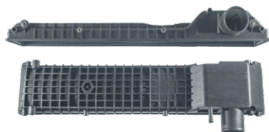
11729 Caterpillar / Valtra / BH 180 / Massey New Holland (bocal lado) (retorno fino)
